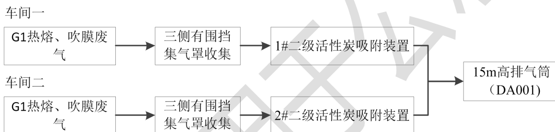
图4-2废气处理工艺示意图
