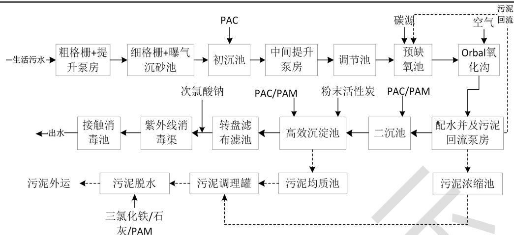
附图 4-1 常州郑陆污水处理有限公司污水处理工艺图
