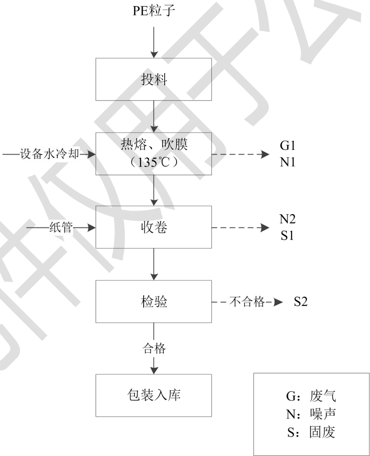
图 2-3 生产工艺流程及产污节点图
