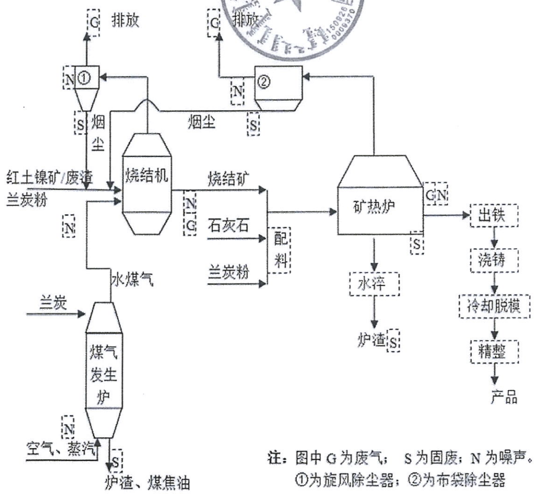
生产工艺流程及产污环节图
