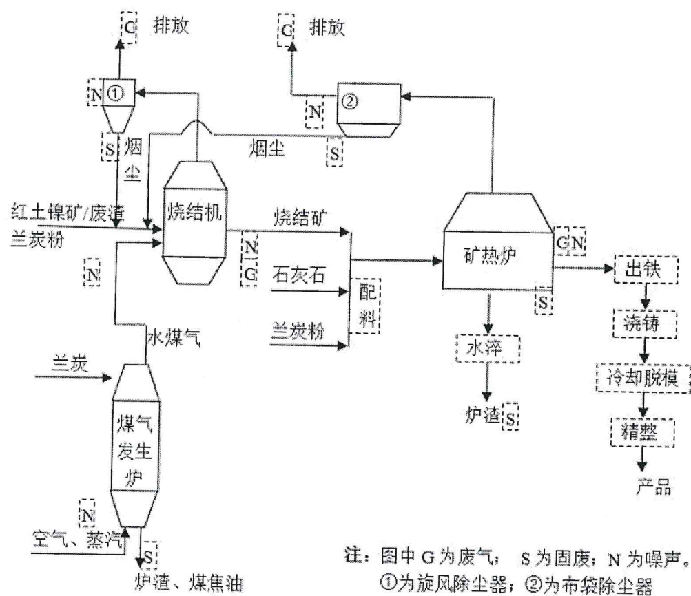
生产工艺流程及产污环节图
